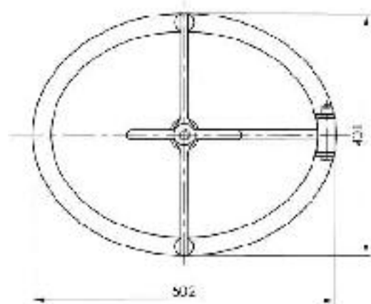
Art. 6008
